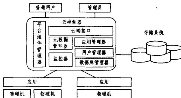
图 5 SaaS 的体系结构图
